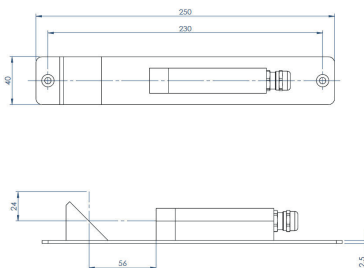
Capteur de niveau à ultrasons CSA
